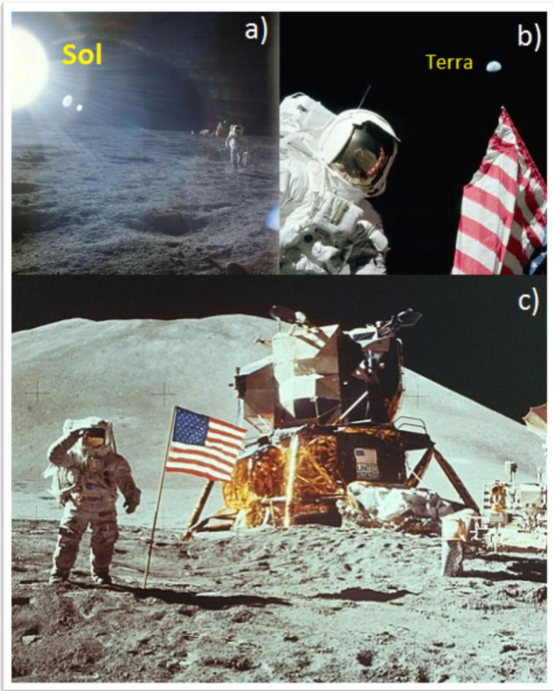
a) A luz direta do Sol espalhada na lente da câmera fotográfica e b) a Terra vistos da Lua pelos astronautas americanos. c) Paisagem lunar iluminada pela luz solar e o fundo escuro do espaço.
